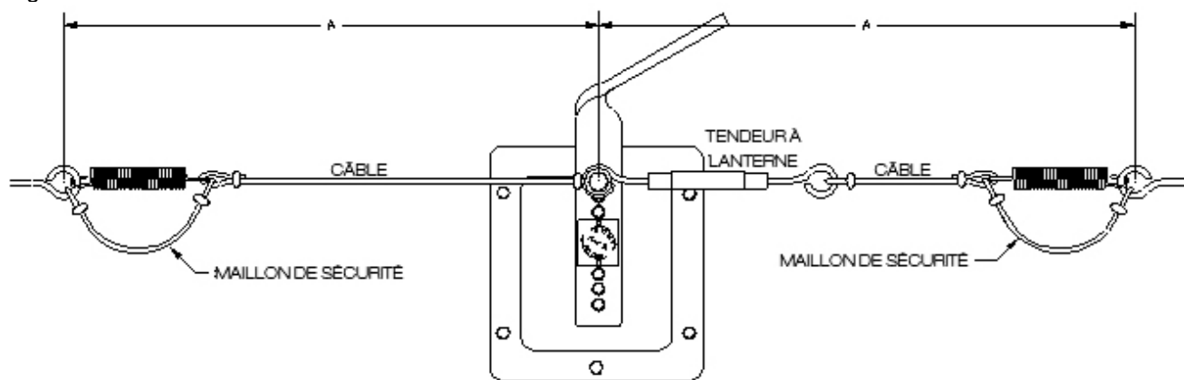
Figure 4 : Ressort de câble
